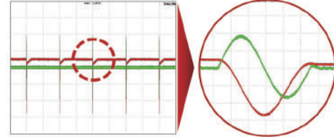
▲ 출력 펄스 정상 파형
