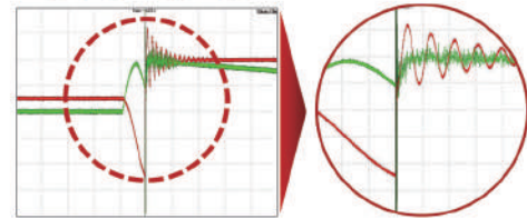
▲ Spark발생 후 출력 IGBT차단 파형
